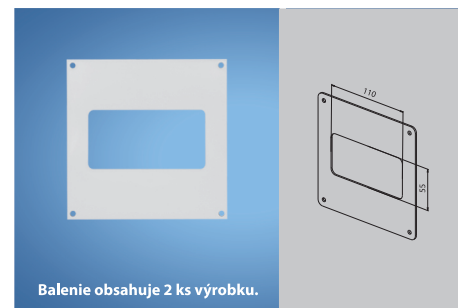
Príruba nástenná
