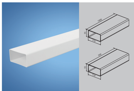
Plochý kanál
